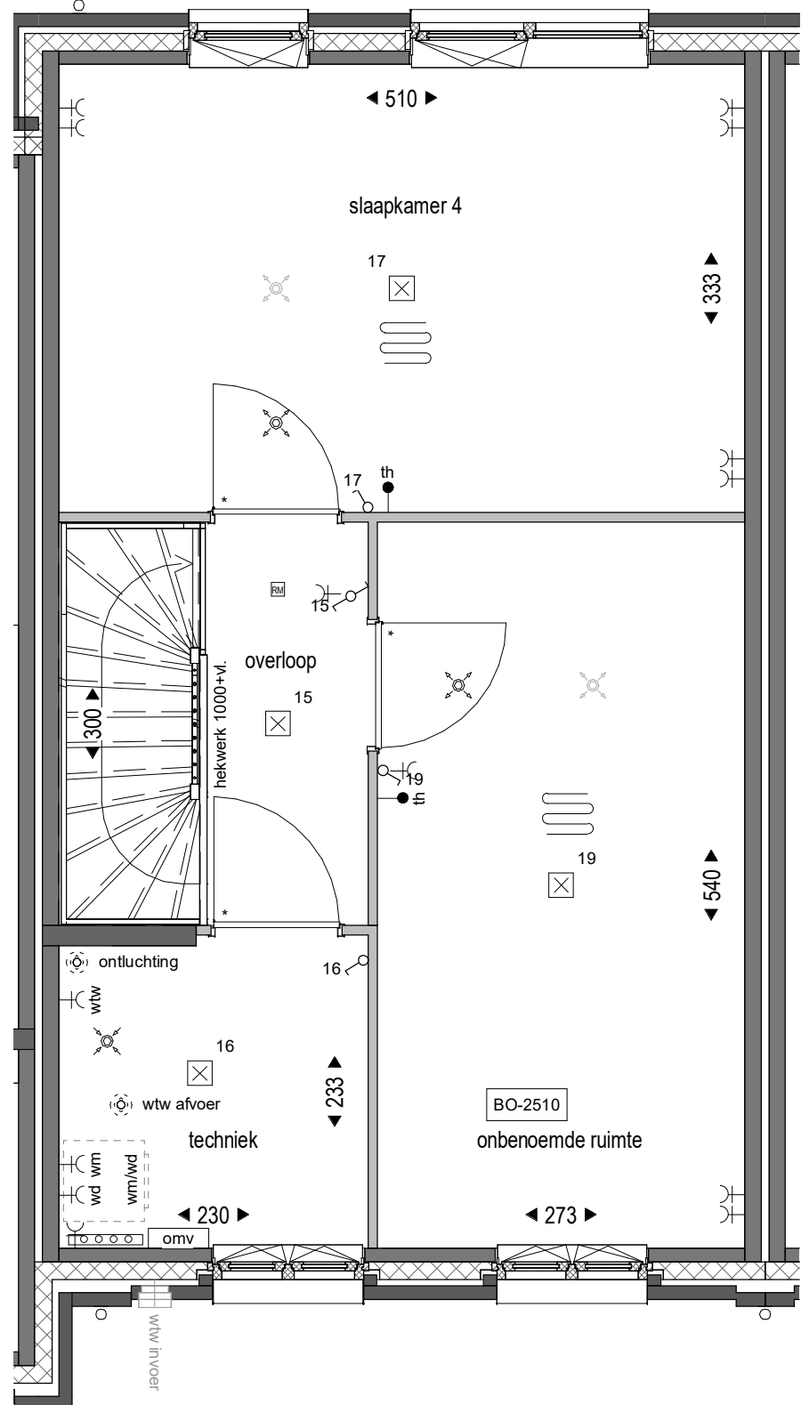
Type H3 VERDIEPING 2 - BO-2510 indeling zolder met onbenoemde ruimte
