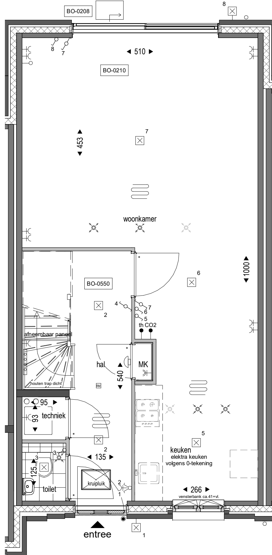
Type H3 BEGANE GROND - BO-0208 schuifrichting schuifpui wijzigen - BO-0210 uitbouw achtergevel 1,2m - BO-0550 hal vergroting (alleen i.c.m. uitbouw 1,2m/2,4m)
