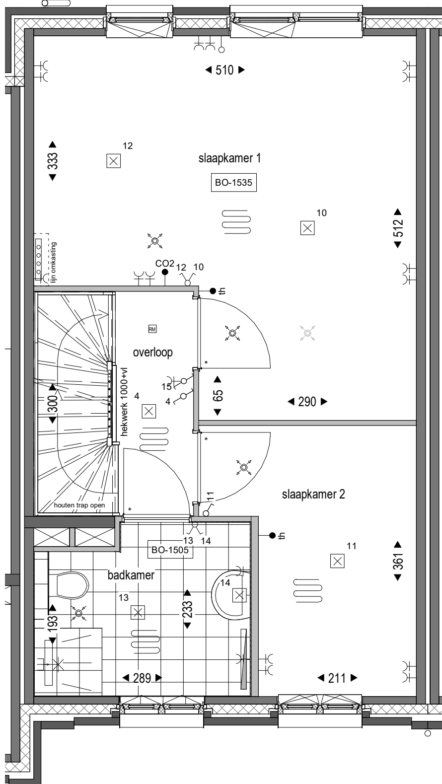
Type H3 VERDIEPING 1 - BO-1535 samenvoegen slaapkamer 1 en 3 - BO-1505 vergroten badkamer (60cm) optie 2
