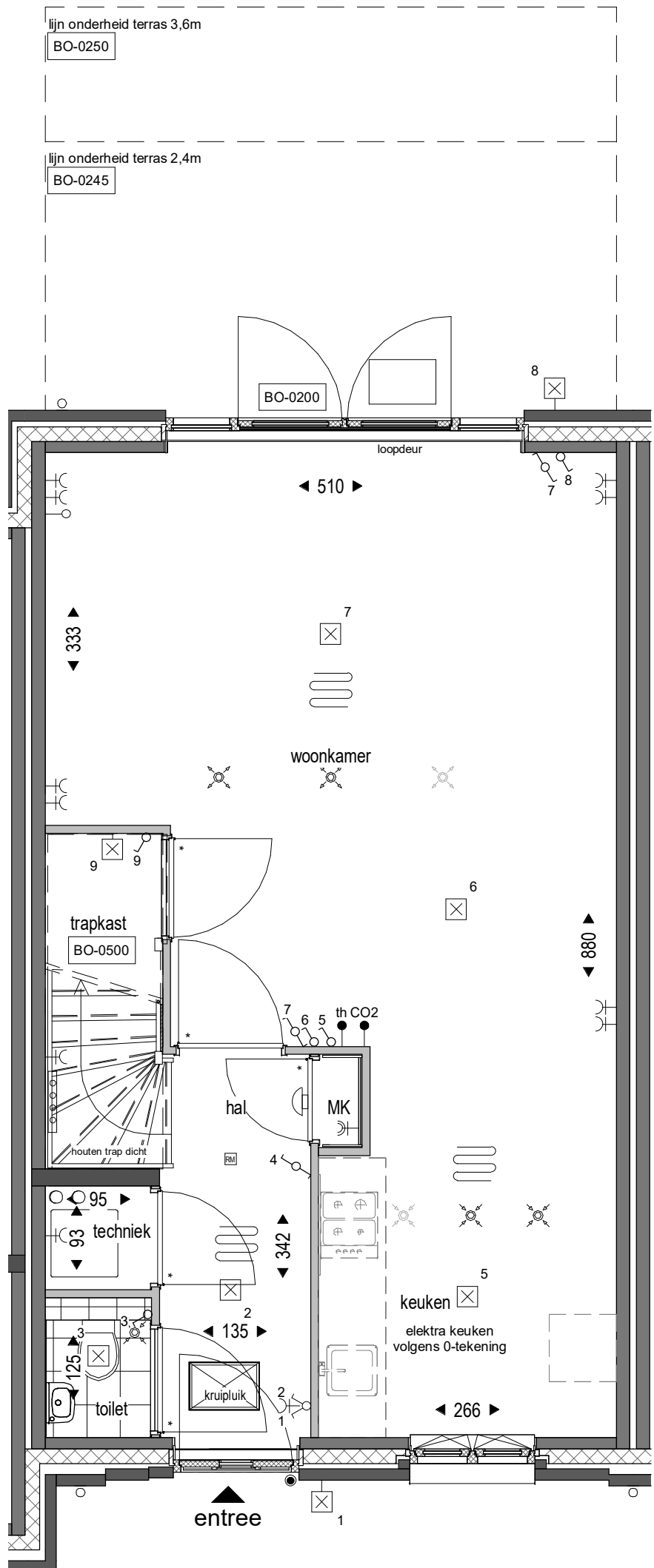
Type H3 BEGANE GROND - BO-0200 tuindeuren in achtergevel - BO-0500 trapkast - BO-0245 onderheid terras 2,4m - BO-0250 onderheid terras 3,6m
