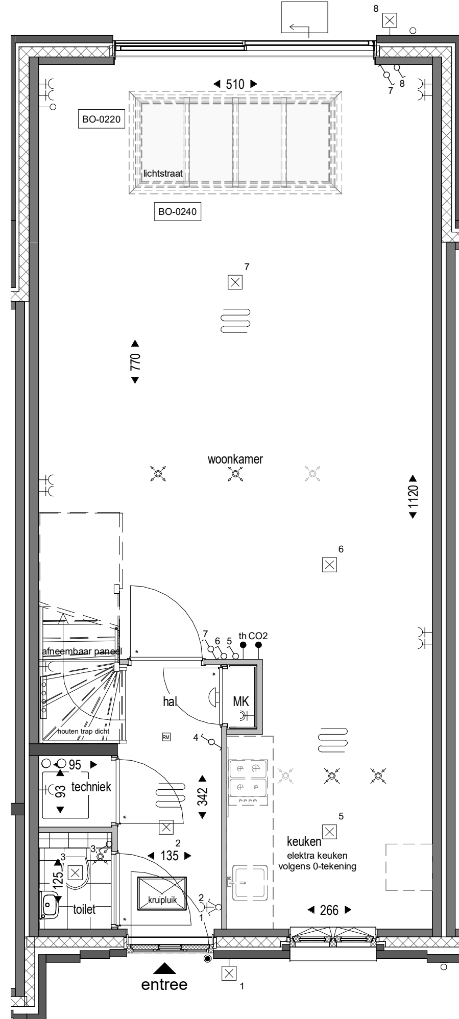
Type H3 BEGANE GROND - BO-0220 uitbouw achtergevel 2,4m - BO-0240 lichtstraat (alleen i.c.m. uitbouw 2,4m)
