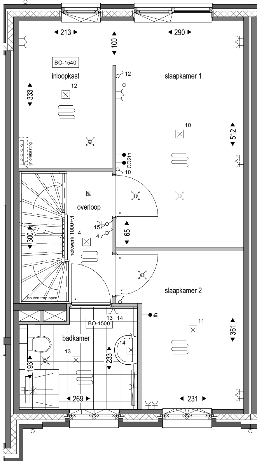
Type H3 VERDIEPING 1 - BO-1540 inloopkast creëren van slaapkamer 3 - BO-1500 vergroten badkamer (40cm) optie 1
