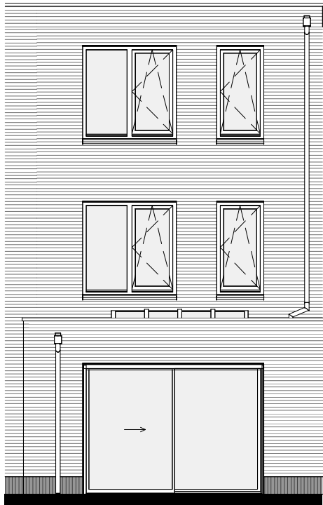
Type H3 ACHTERGEVEL - BO-0220 uitbouw achtergevel 2,4m - BO-0240 lichtstraat (alleen i.c.m. uitbouw 2,4m)
