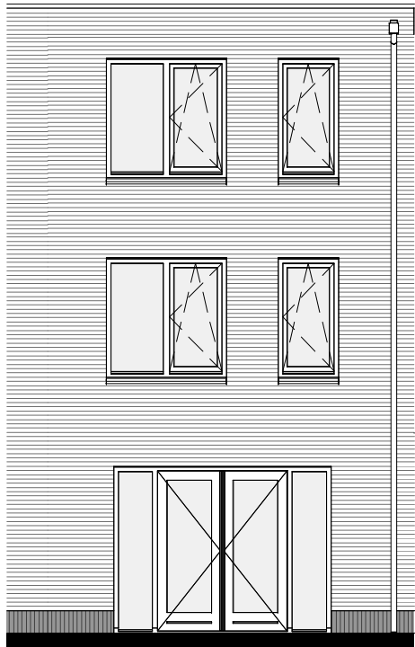
Type H3 ACHTERGEVEL - BO-0200 tuindeuren in achtergevel
