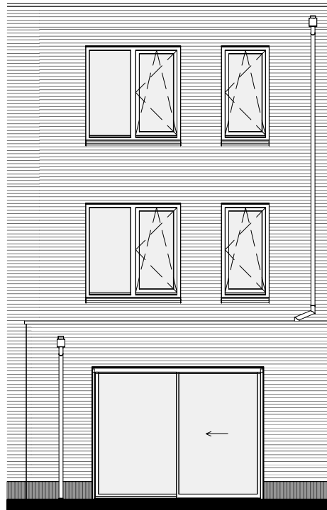
Type H3 ACHTERGEVEL - BO-0208 schuifrichting schuifpui wijzigen - BO-0210 uitbouw achtergevel 1,2m
