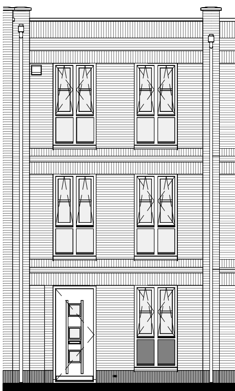
Type H3 VOORGEVEL - BO-0005 onderzijde kozijn dichtzetten met geëmailleerd glas
