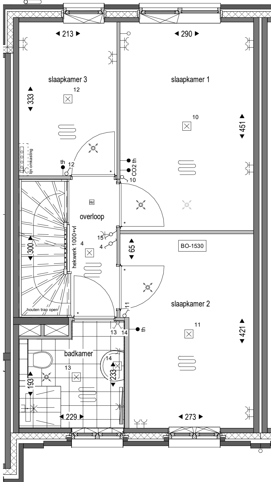
Type H3 VERDIEPING 1 - BO-1530 wand tussen slaapkamer 1 en 2 verplaatsen
